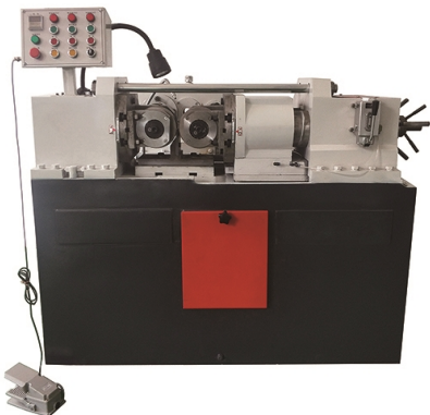
两轴滚丝机
